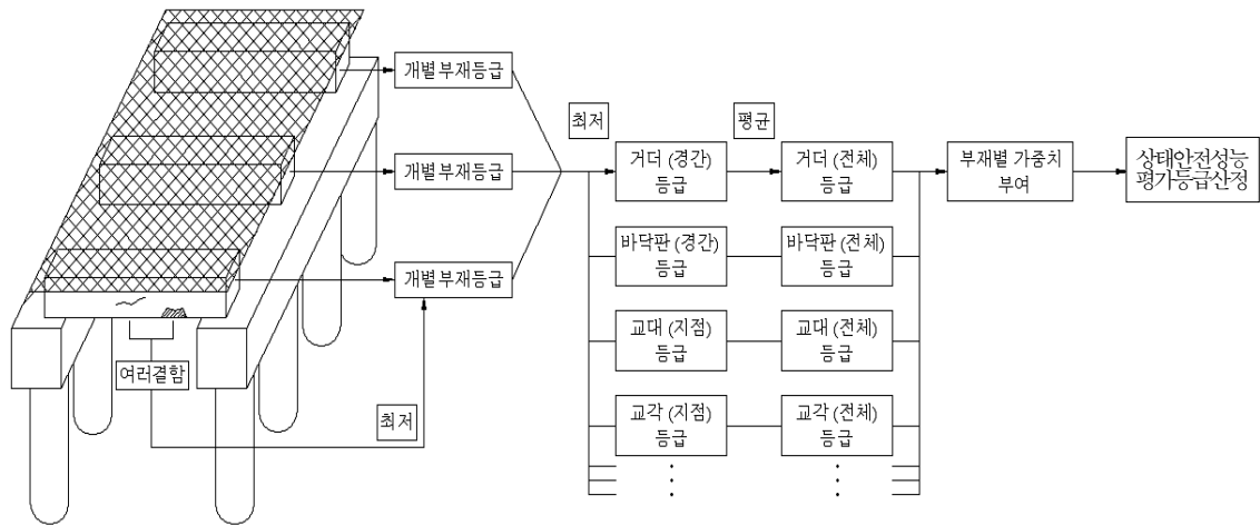
[그림 1.34] 전체 교량의 상태안전성능 결과 산정 예
