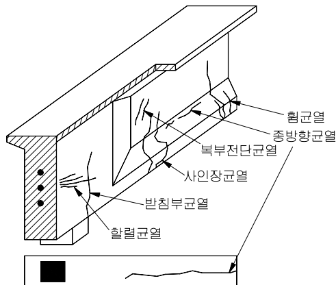
[그림 1.7] PSC 거더의 조사부위
