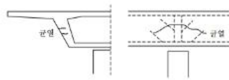
[그림 1.10] PSC 박스거더의 균열
