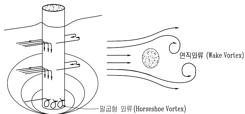
[그림 1.19] 월형기초의 국부세굴
