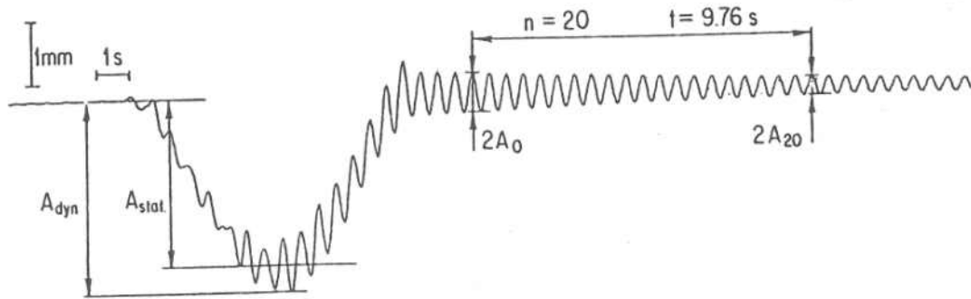
[그림 1.28] 변위 이력곡선의 예
