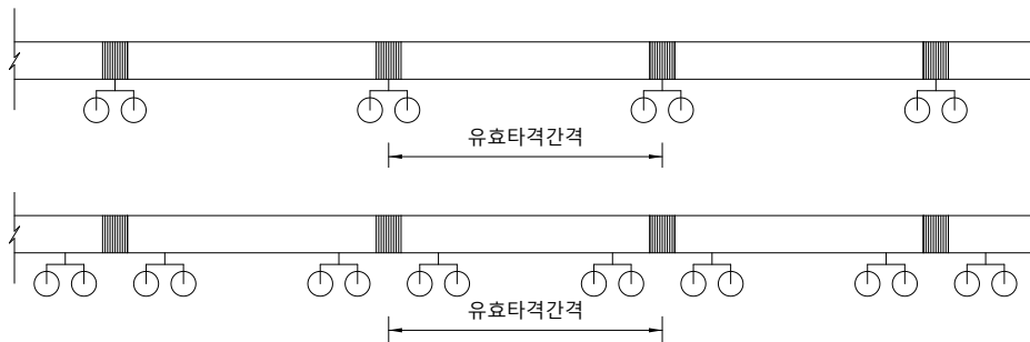
[그림 1.29] 운행열차에 대한 유효타격간격 결정방법
