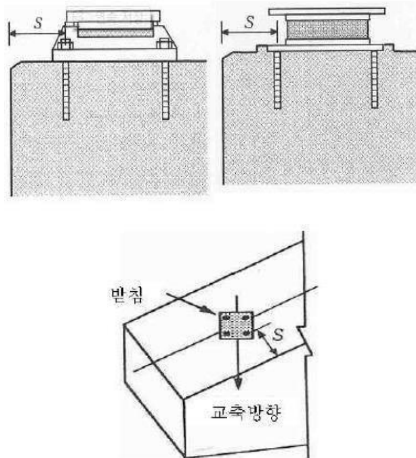
[그림 1.21] 교량받침의 연단거리
